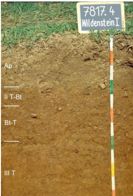
Tief entwickelte erodierte Terra fusca-Parabraunerde aus lösslehmreichen Fließberden über periglazial umgelagertem Höhenschotter-Verwitterungston
