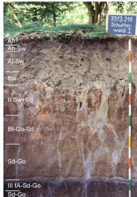
Parabraunerde-Gley-Pseudogley aus spätwürmzeitlichem Hochflutsediment der Kinzig (x41)
