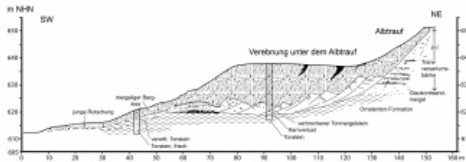
Schnitt durch eine Hangschutt-Terrasse unterhalb des Albraufs
