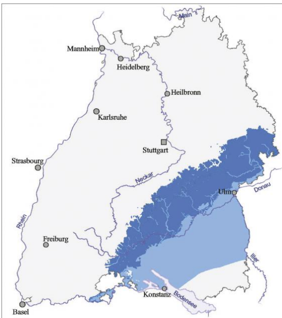
Verbreitung des Oberjuras in schwäbischer Fazies farbig, Austrich dunkel
