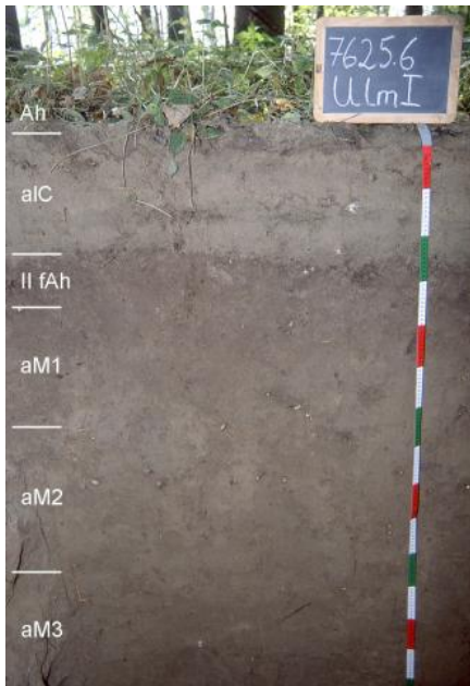
Kalkreicher Brauner Auenboden, von geringmächtiger Auenpararendzina überlagert, aus jungem Hochflutsediment über sandig-schluffigen Auensedimenten auf Illerschotter
