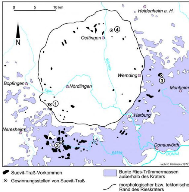
Übersichtskarte mit einer Darstellung der Ausdehnung des Nördlinger Rieskraters und der Verbreitung von Ries- Suevit-Vorkommen und Buntten Riestrümmerrmassen außerhalb des Kraters (nach: Hüttner 1977, verändert). Eingetragen sind wichtige Steinbrüche: (1) Altenbürg, (2) Seelbronn, (3) Otting, (4) Aumühle. Die wichtigen baden-württembergischen Vorkommen befinden sich im Raum Egingen-Hofen-Dunstelkingen (2).
