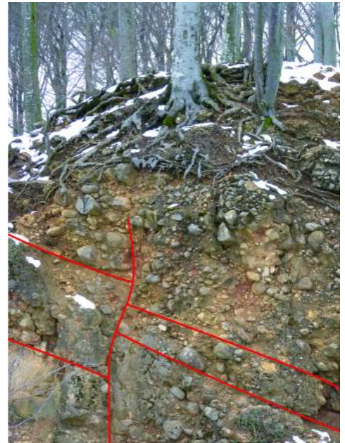
Tertiärkonglomerat an der Schneeberg oberhalb von Ebringen besteht aus Geröllen von Hauptrogenstein.
