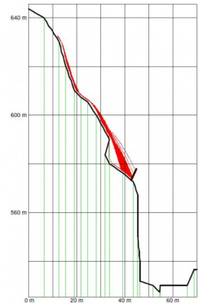
Steinschlagmodellierung am Hohfels
