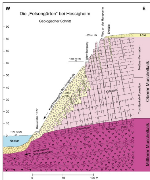
Geologischer Schnitt im Bereich der Felsengärten bei Hessigheim, mit Darstellung der Hangzerreißung im Oberen Muschelkalk und dem Hangkriechen im Bereich der Hangschuttauflage in Folge der Sulfatauslaugung durch den Neckar im Mittleren Muschelkalk
