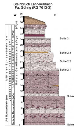
Säulenprofil des aktuellen Abbaus im Steinbruch Lahr-Kuhbach
