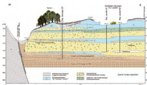
Geologischer Schnitt durch das Vorkommen von Süßwasserkalken bei Gaugingen
