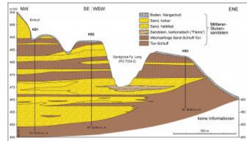
Geologischer Schnitt durch die Stubensandstein-Schichten bei Gschwend
