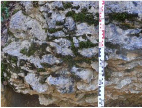
Dünnbankiger, flaserig-knaueriger Kalkstein. Einzelne Mergelsteinlagen treten in der Böschung als Hohlkehle zurück
