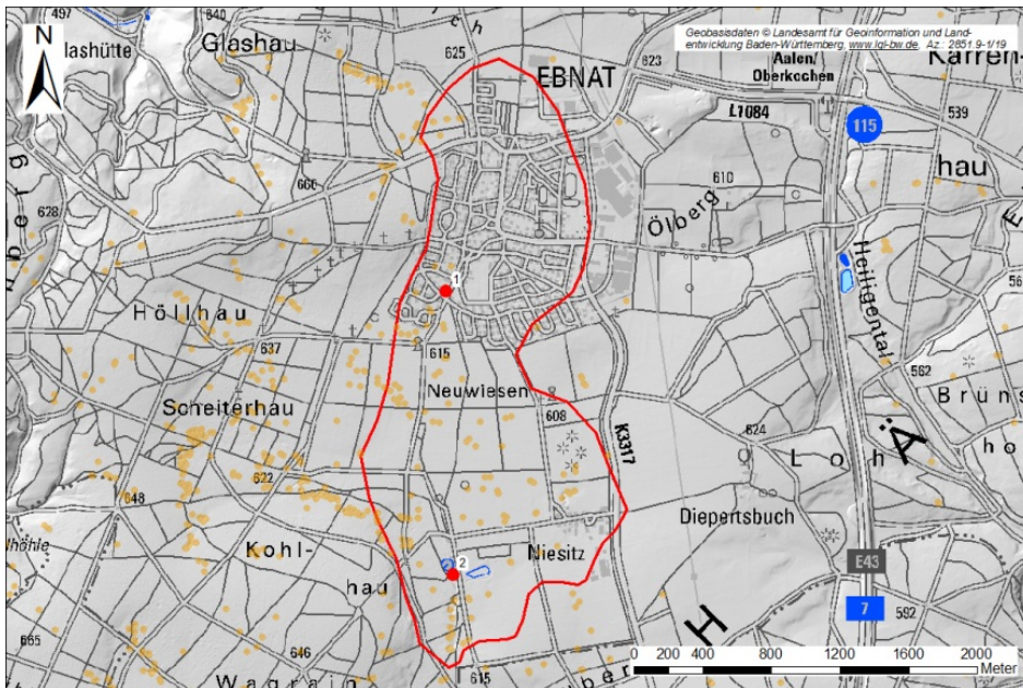
Lage der Ebnater Karstwanne (rote Umrandung; nach Groschopf & Kobler, 1974) mit Verkarstungsstrukturen nach IGHK50 (orange Punkte) sowie Lage des Hexenlochs (1) und Kohlhau-Schachts (2) (rote Kreise).
