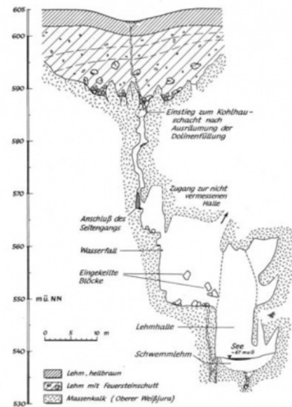
Schnitt durch Doline und Kohlhou-Schacht bei Ebnat (Grafik: Groschopf & Kobler 1974)
