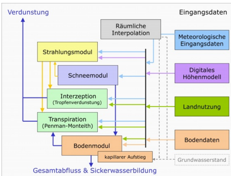
Module des Modells GWN-BW zur prozessbasierten Modellierung der Grundwasserneubildung (Grafik: www.hydrosconsult.com/hydrologie/bodenwasserhaushalt/ )
