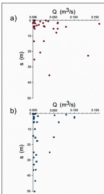
Leistungsdiagramme für Entnahmebrunnen im Oberjura-Karstgrundwasserleiter der Ostalb (Grafik: HGK, 2002)
