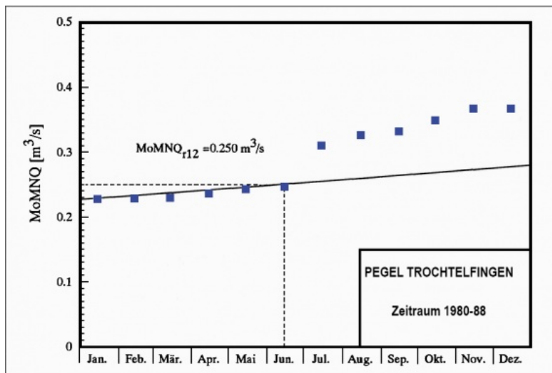
Ermittlung des langfristigen Karstwasseranteils im Abfluss der Seckach am ehemaligen Pegel Trochtelfingen (MoMNQr12-Verfahren nach Villinger, 1981b, aus Jentsch & Franz, 1999).
