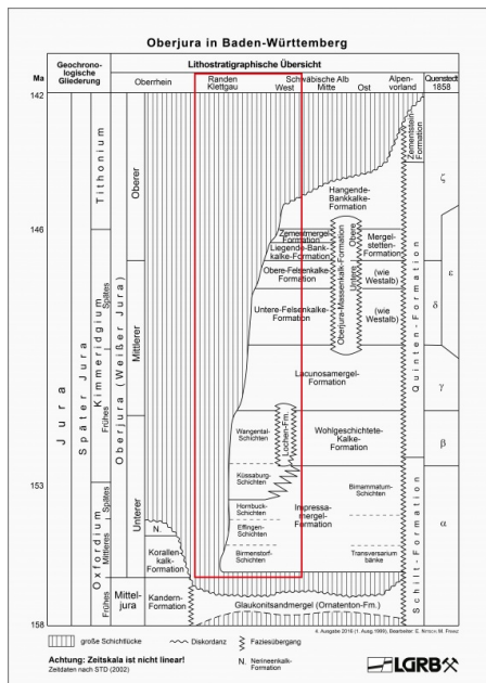
Schichtenfolge des Oberjuras in der Hydrogeologischen Region Westalb, Hegualb und Klettgau
