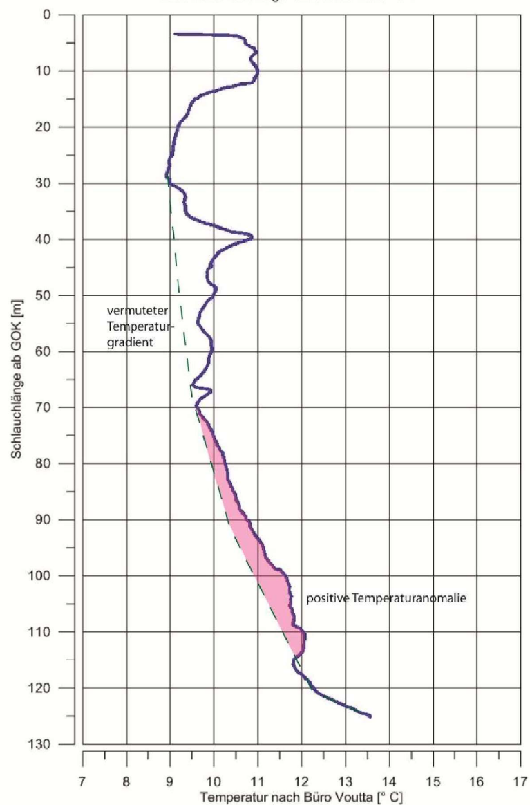
Ruhetemperaturprofil; [REDACTED], Böblingen; EWS 1
