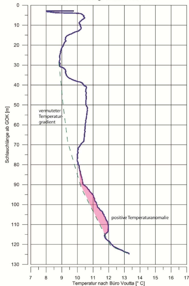
Ruhetemperaturprofil; [REDACTED], Böblingen; EWS 2
